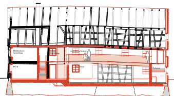
SCHNITT
